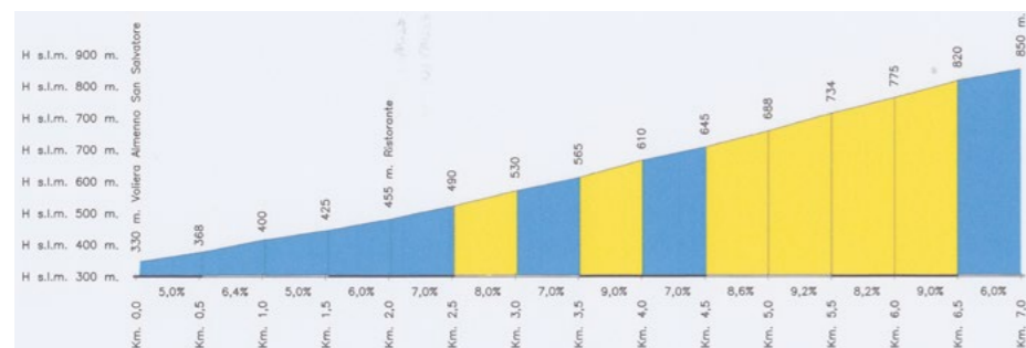
Altimetria della salita in Roncola
